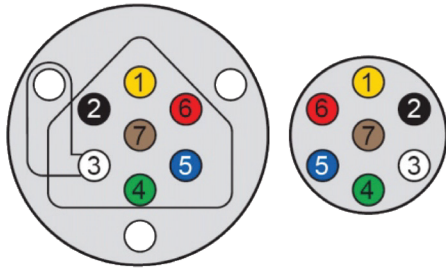
7 Pole Socket
